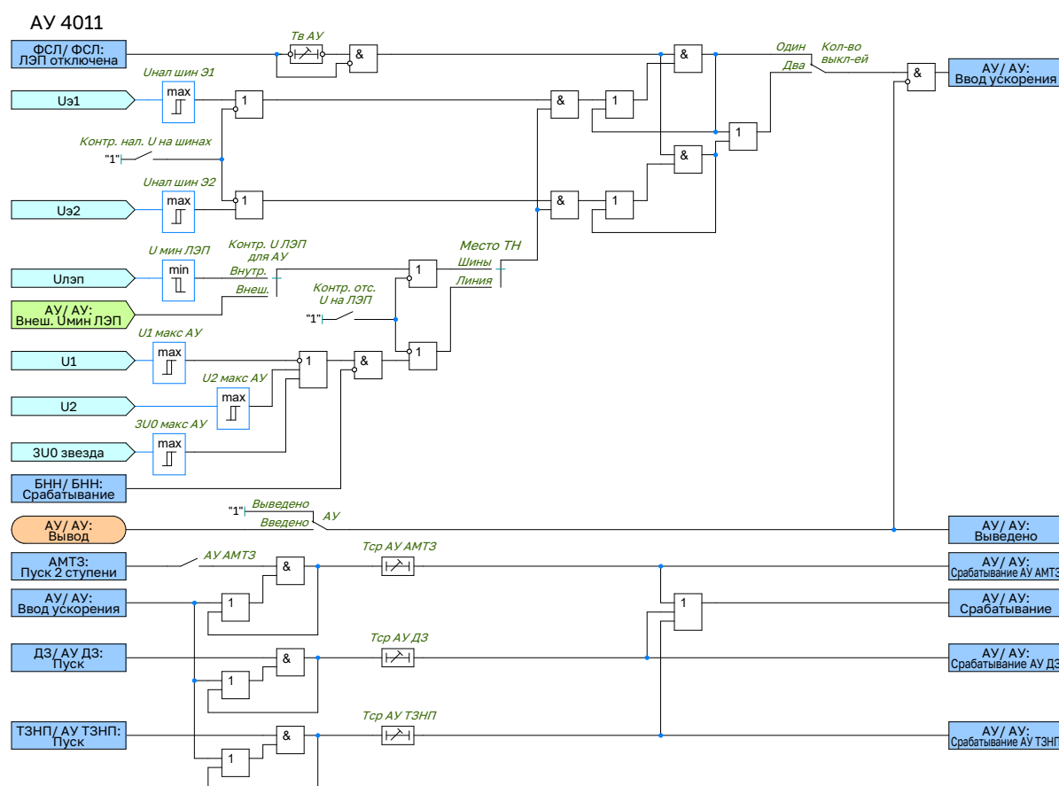
Рисунок 2.37 – Функциональная схема АУ
